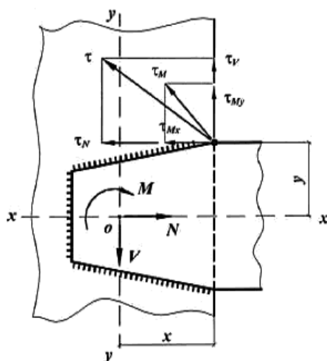
Рисунок 21 - Расчетная схема сварного соединения
